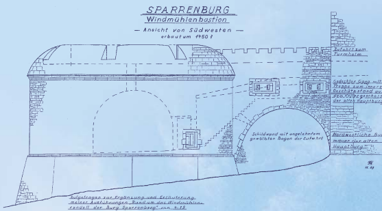
Dibujo reconstruido de la rotonda del molino de aire (construido en el siglo 15), F.K. Wittenborn 1989
