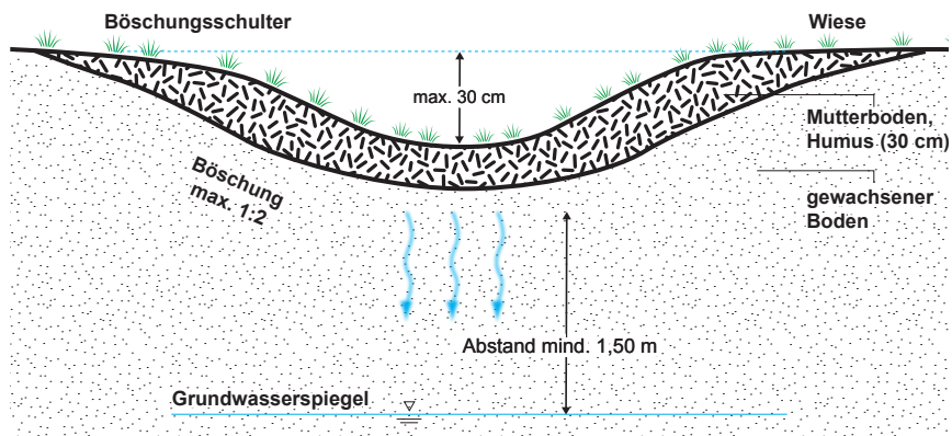
Prinzipische Skizze Mulden-Versickerung
