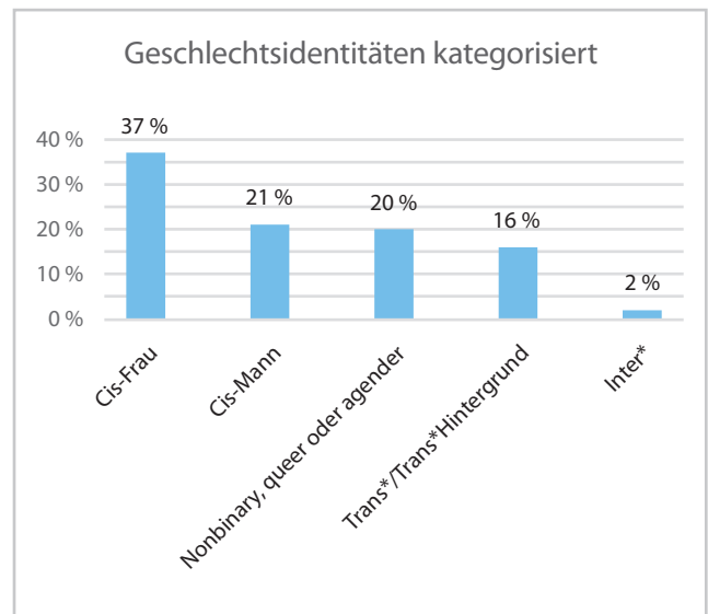
Abb. 4: Geschlechtsidentitäten kategorisiert (n = 830)
