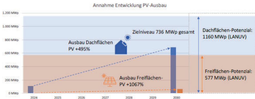
Abbildung 32 Entwicklungspfad des PV-Ausbaus im Zielszenario (Grafik: Gertec GmbH)
